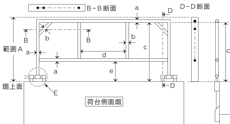
【積載物飛散防止装置：図2-1】
