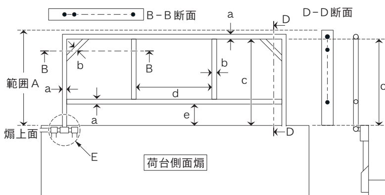
【積載物飛散防止装置：図2-2】
