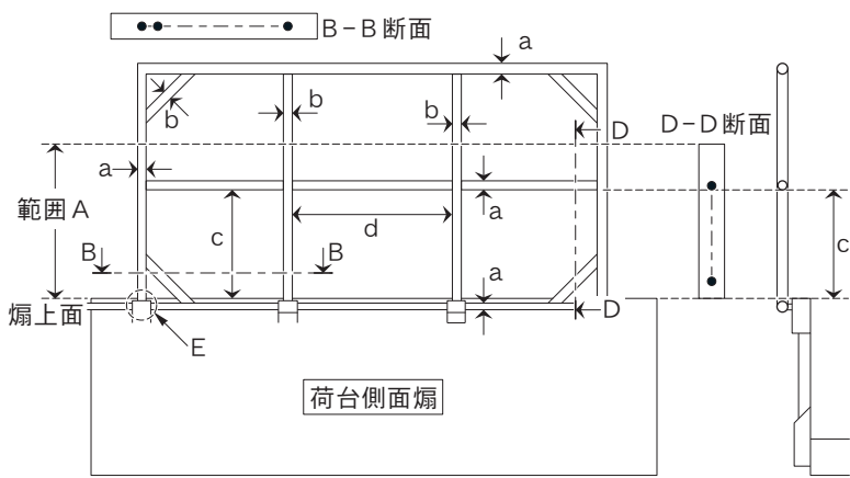
【積載物飛散防止装置：図1-2】
